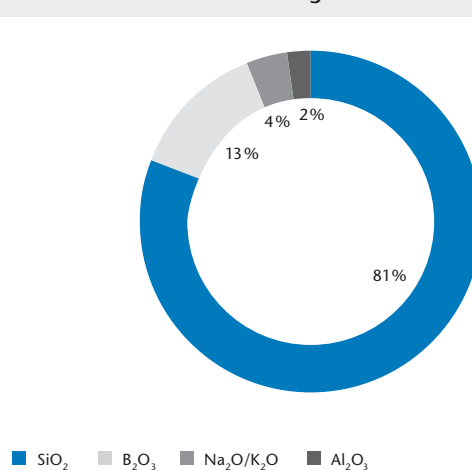
Chemische Bestandteile von BOROFLOAT® 33.
